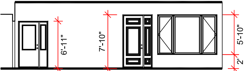
8 4 Élévation # 8
